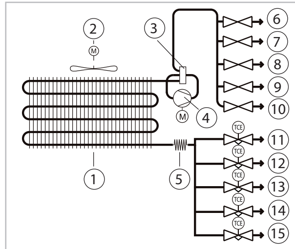
Abb. 2: Schema Kältekreis
