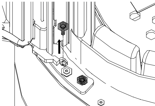
Abb. 58: Schrauben unten
