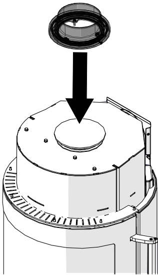
Abb. 36: Drehrauchrohrstutzen montieren
