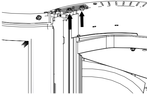
Abb. 46: Türscharniere einstellen
