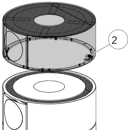
Abb. 19: Aufsatzbox aufsetzen
