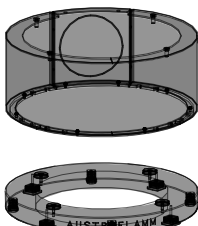
Abb. 32: Sockelbox mit Holzsockel
