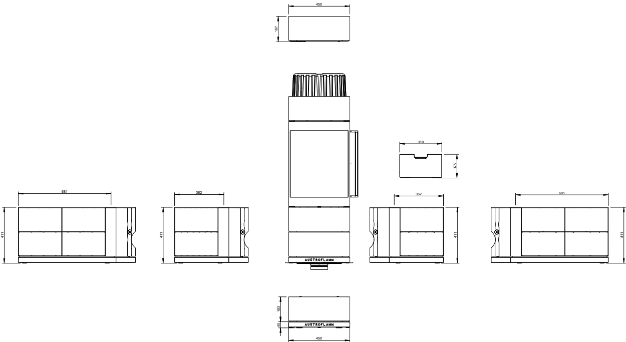
Abb. 3: Abmessungen Beistellboxen
