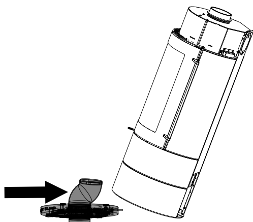
Abb. 38: Kaminofen kippen
