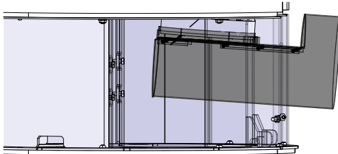
Abb. 31: Zuluftadapter montieren
