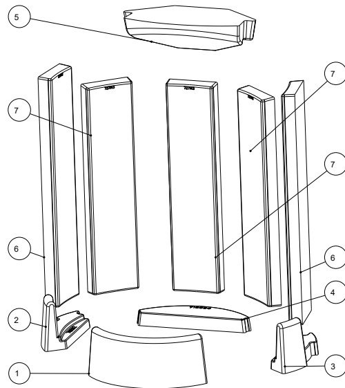
Abb. 16: Keramott einbauen
