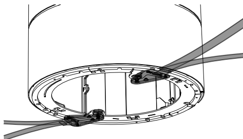
Abb. 9: Transporthilfe
