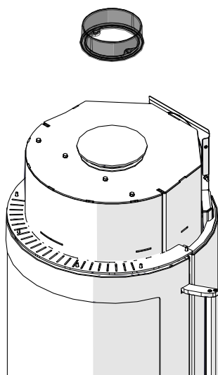
Abb. 35: Rauchrohrstutzen abmontieren
