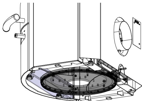
Abb. 22: Drehteller platzieren
