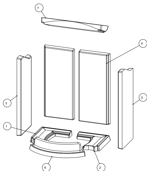
Abb. 15: Keramott einbauen
