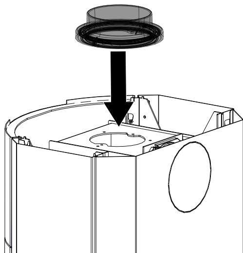
Abb. 19: Drehrauchrohrstutzen montieren
