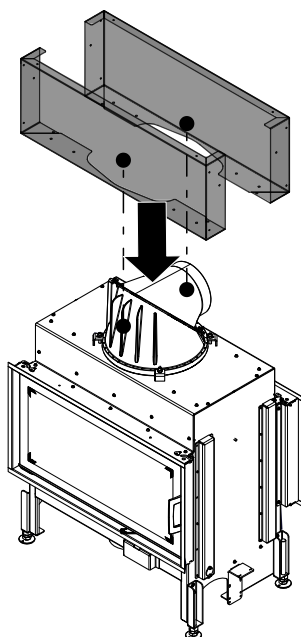
Abb. 76: KV-Wand oben (vorne + hinten) montieren
