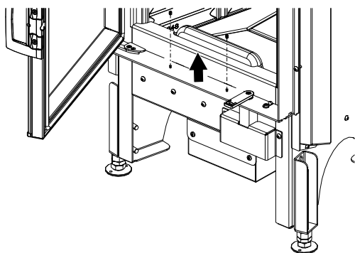
Abb. 83: Bolzen unten rausdrehen
