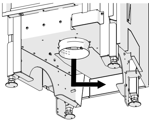
Abb. 5: Verbrennungsluftstutzen
