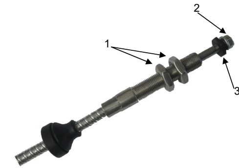
Abb. 56: Steuerungseinheit einbauen
