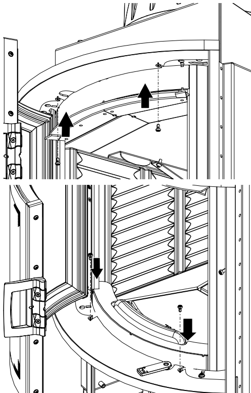
Abb. 88: Designrahmen befestigen
