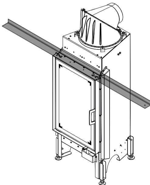
Abb. 96: Tragrahmen montieren
