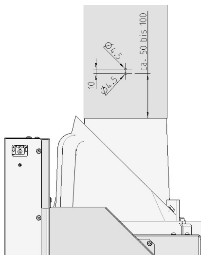
Abb. 49: Bohrschema-Rauchrohr
