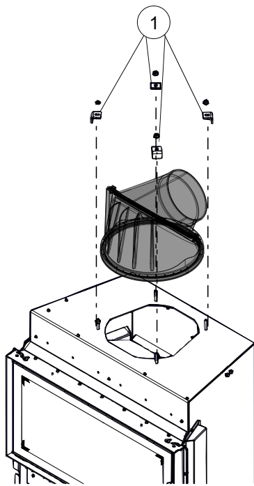
Abb. 43: Rauchsammler abmontieren
