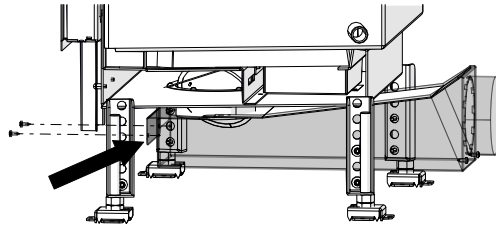
Abb. 40: Flachknie anbringen
