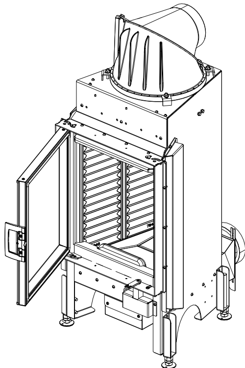
Abb. 81: Tür öffnen
