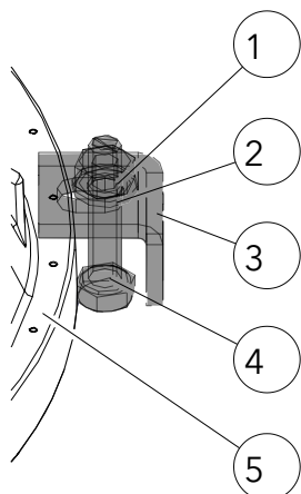
Abb. 38: Abgassammler montieren
