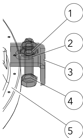
Abb. 45: Abgassammler montieren
