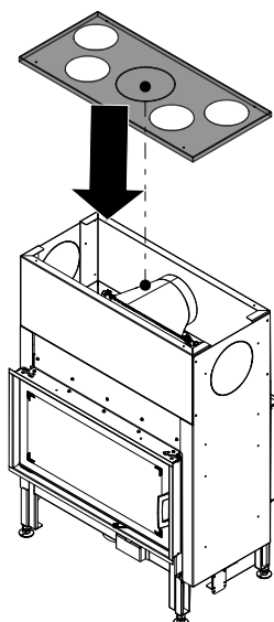
Abb. 79: KV-Deckel montieren
