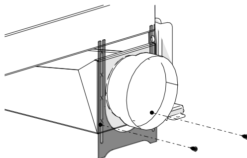
Abb. 41: Befestigung montieren
