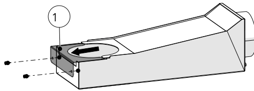
Abb. 39: Schrauben lösen
