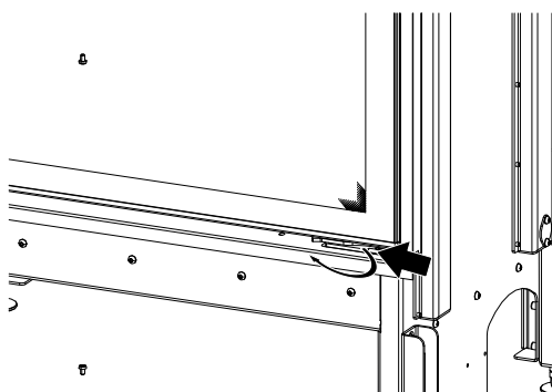
Abb. 93: Feder aufmachen
