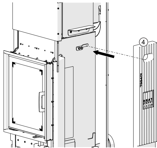
Abb. 28: HMS-Stein anbringen
