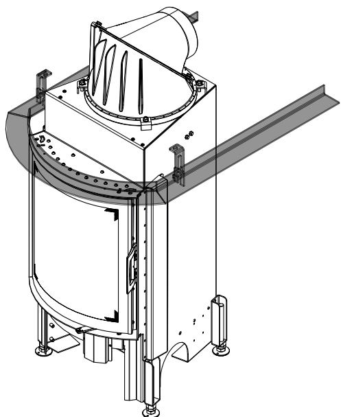
Abb. 97: Tragrahmen montieren
