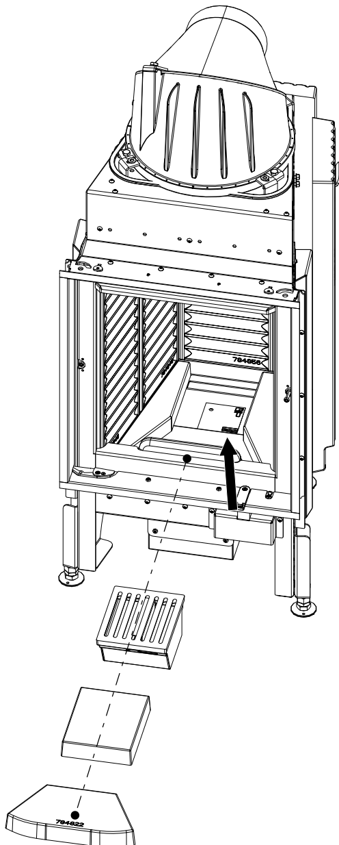
Abb. 98: Aschenkasten einlegen
