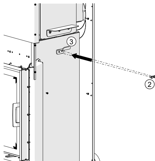
Abb. 27: HMS-Halter montieren
