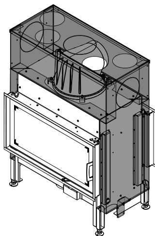
Abb. 80: KVM montiert
