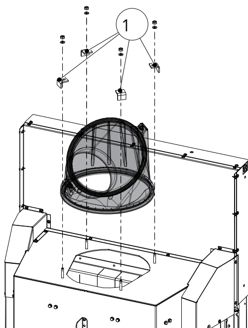
Abb. 36: Rauchsammler abmontieren
