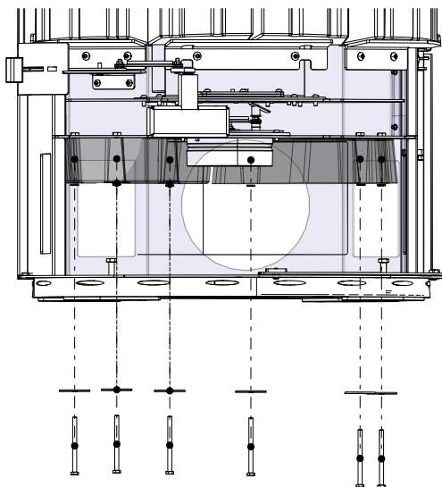
Abb. 9: HMS-Steine unten montieren
