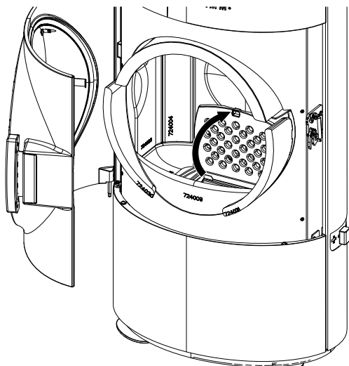
Abb. 33: Rost hochklappen
