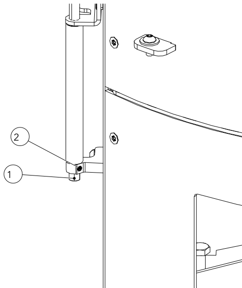
Abb. 29: Türschließkraft einstellen
