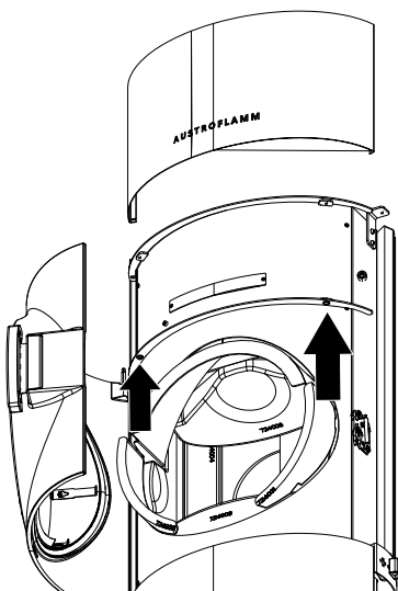
Abb. 22: obere vordere Verkleidung demontieren
