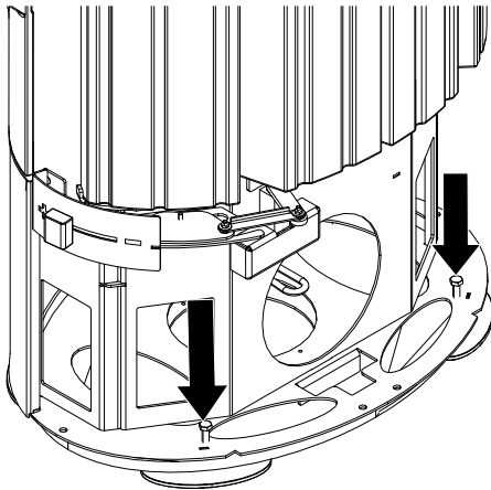
Abb. 20: Kaminofen ausrichten
