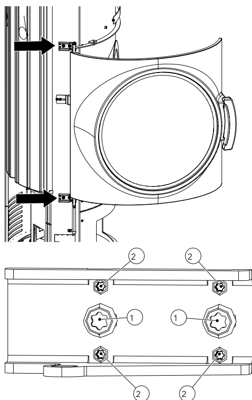
Abb. 24: Türeinstellschrauben
