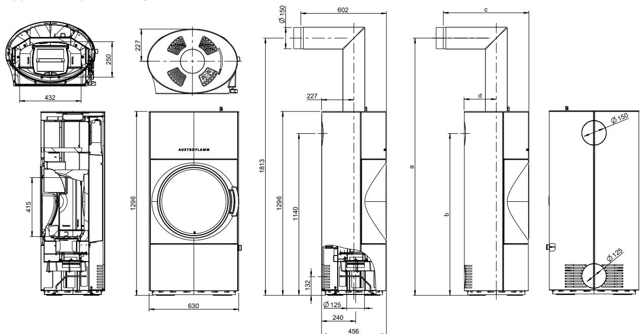
Abb. 2: Abmessungen Grundgerät
