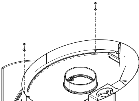
Abb. 21: vordere Verkleidung oben demontieren
