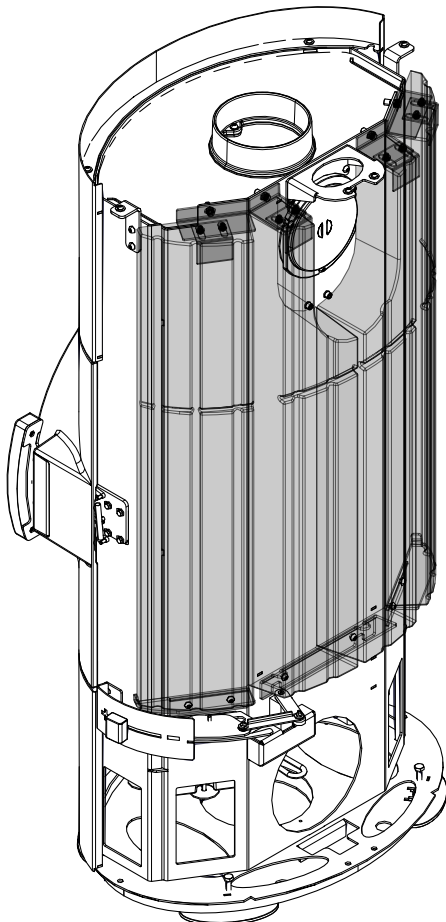
Abb. 8: HMS montieren
