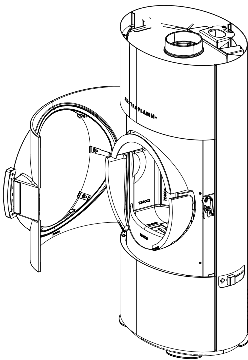
Abb. 27: Tür öffnen
