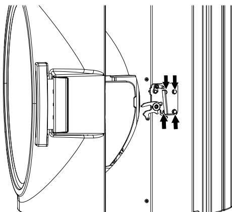
Abb. 26: Türverschluss einstellen
