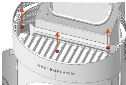
Abb. 34: Befestigungsschrauben abschrauben
