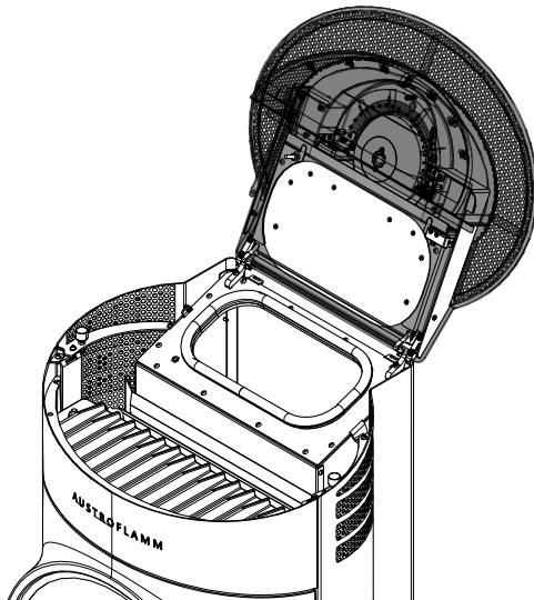
Abb. 33: Revisionsdeckel aufklappen
