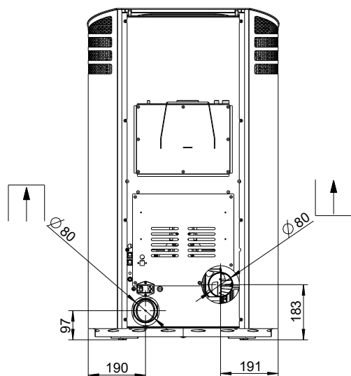
Abb. 11: Anschluss hinten
