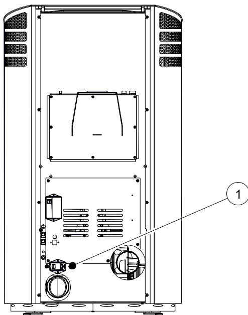
Abb. 37: Sicherheitstemperaturbegrenzer
