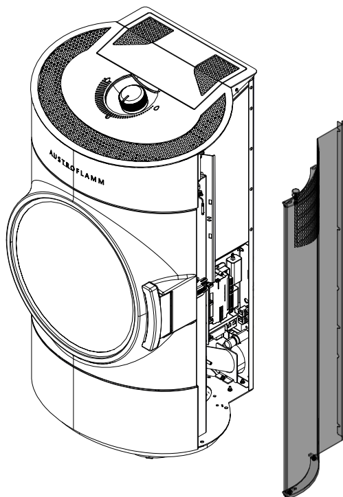
Abb. 24: Seitenverkleidung abnehmen
