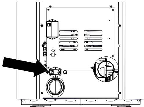
Abb. 38: Sicherungseinschub mit T2,5A-Glasrohrsicherungen
