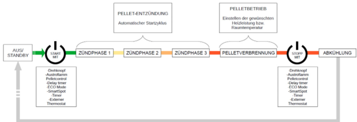
Abb. 17: Funktionsdiagramm
