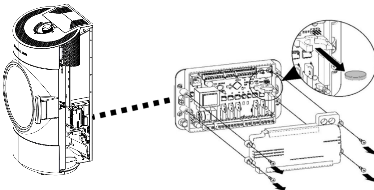
Abb. 25: Speicherbatterie tauschen
