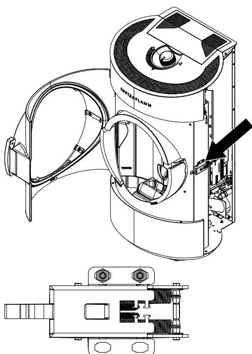
Abb. 23: Türverschluss einstellen
